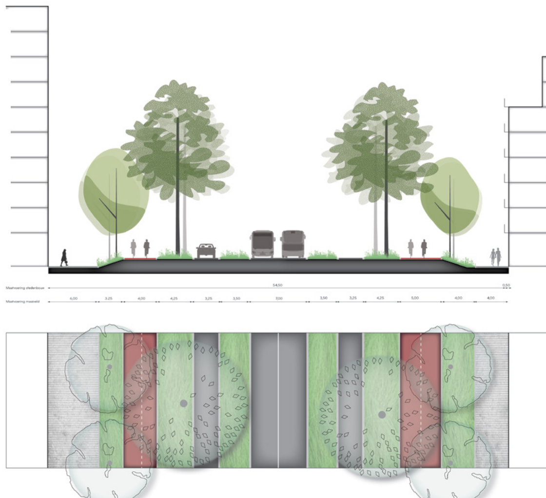
Profiel Koningin Wilhelminalaan
