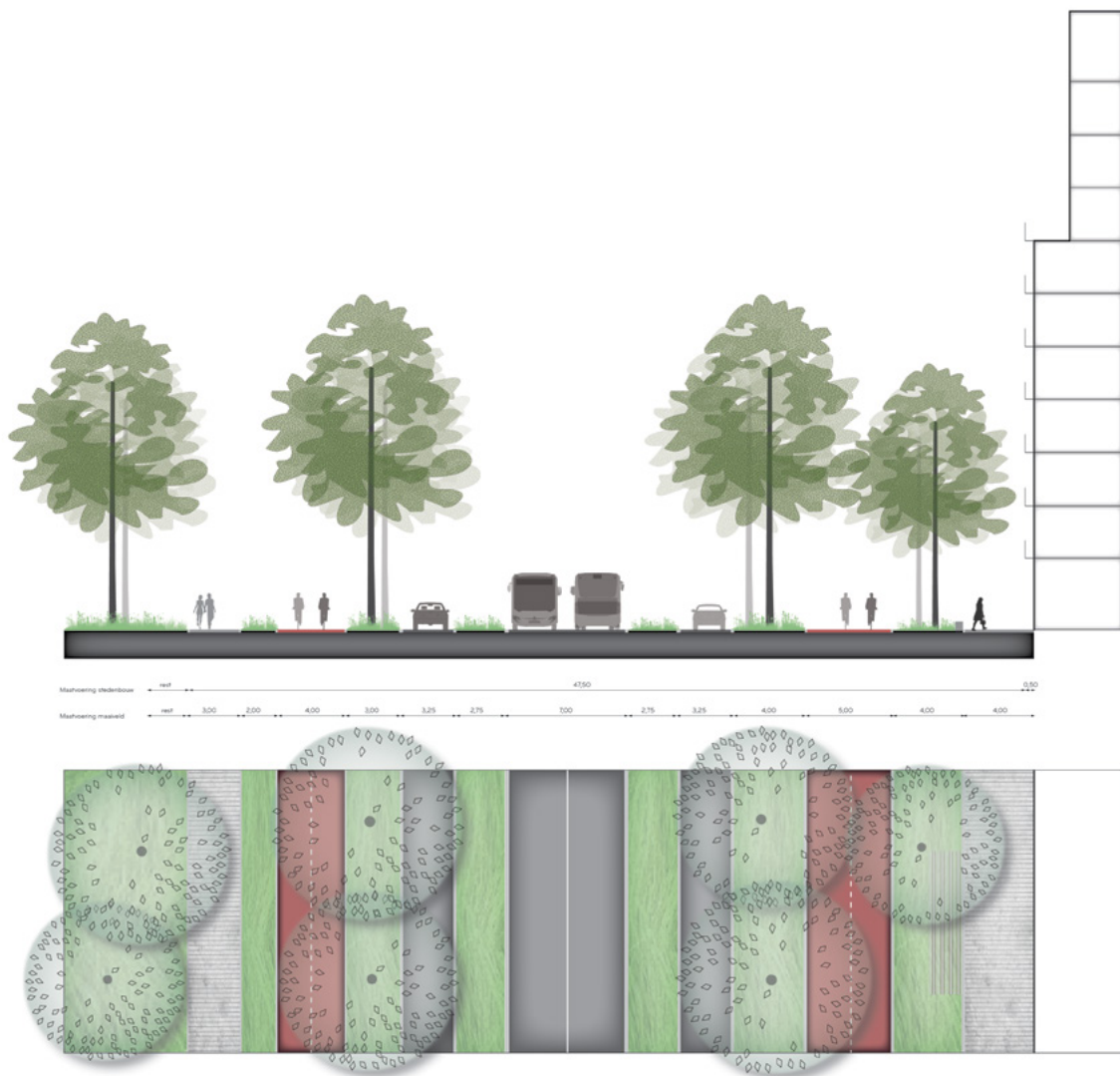
Het profiel van de Europalaan
